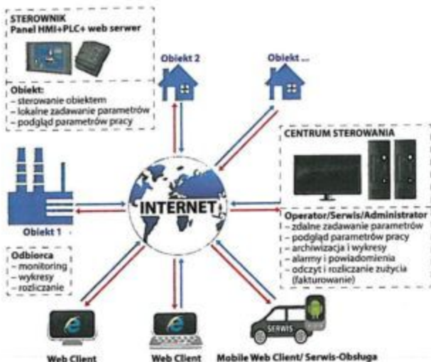
Rys. 2. Koncepcja sterowania obiektami z użyciem Smart Grid
